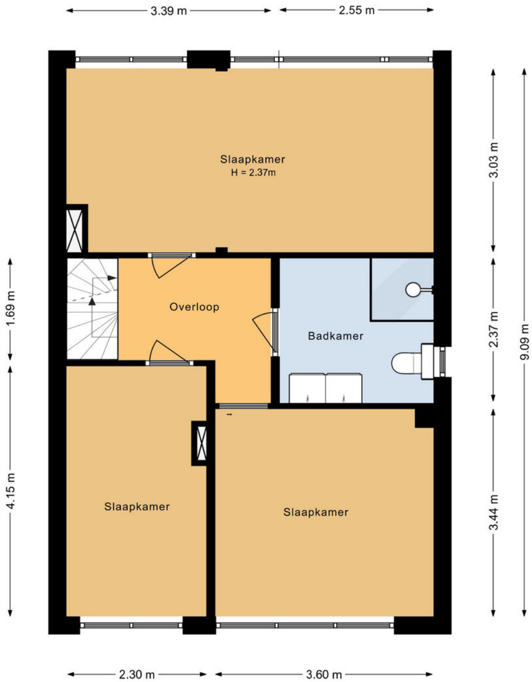
Eerste verdieping Beatrixlaan 17
